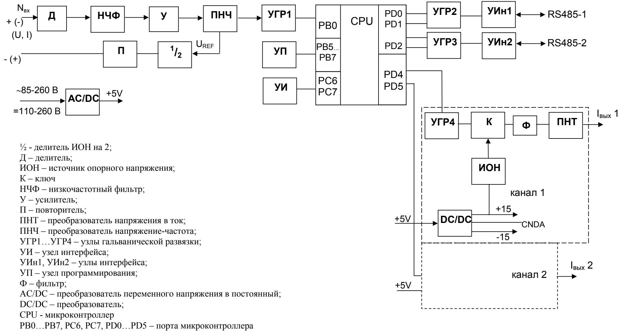
Рисунок Б.1 – Структурная схема преобразователя E856ЭЛ, имеющих исполнения с интерфейсами
