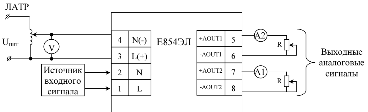
Рисунок В.1 – Схема подключения преобразователя E854ЭЛ, имеющего исполнения с интерфейсами
